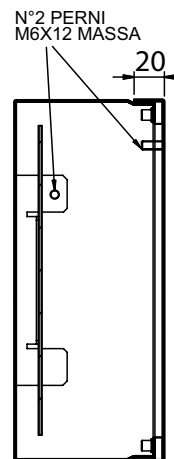
SEZIONE A-A
